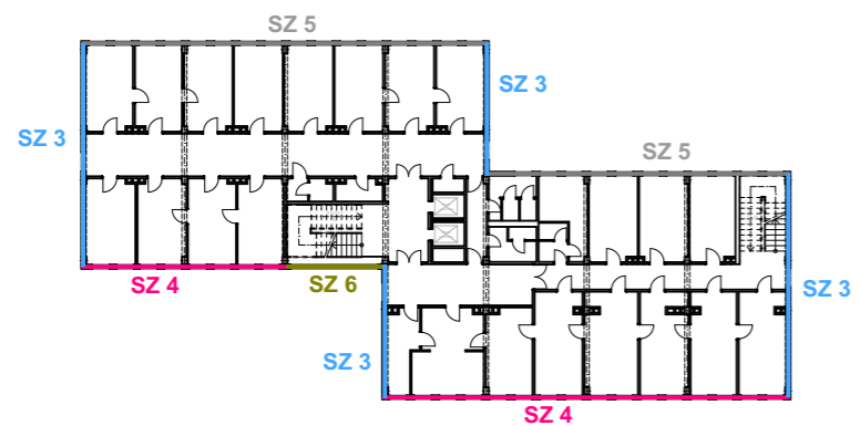
RZUT 2-6 PIĘTRA
